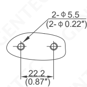
后座安装
